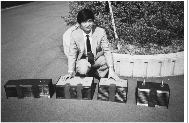
宮川橋に使った免震支承のカットモデル
