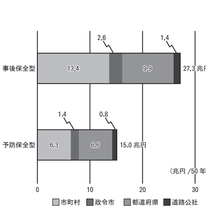
図-2 道路橋の将来メンテナンス費用の全国推計の内訳 ※1 筑波大学堤盛人教授他推計
